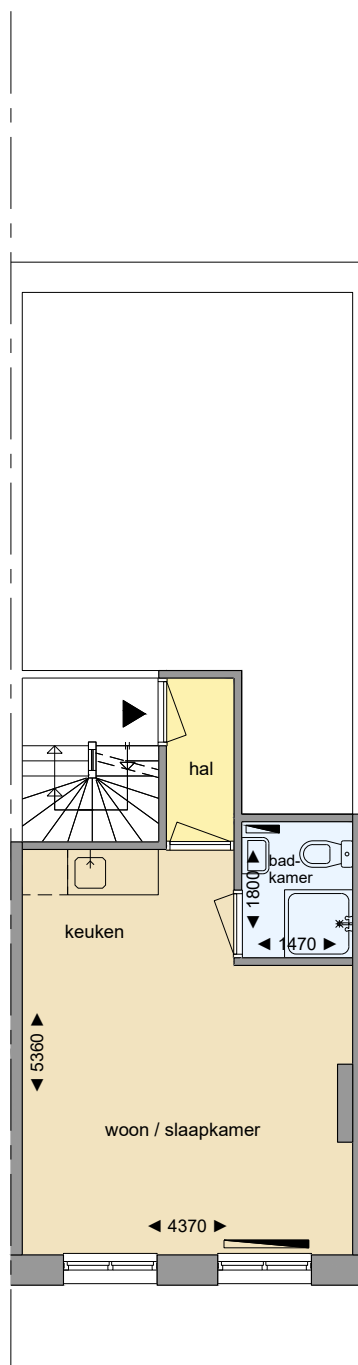
1e en 2e Verdieping schaal 1:100
